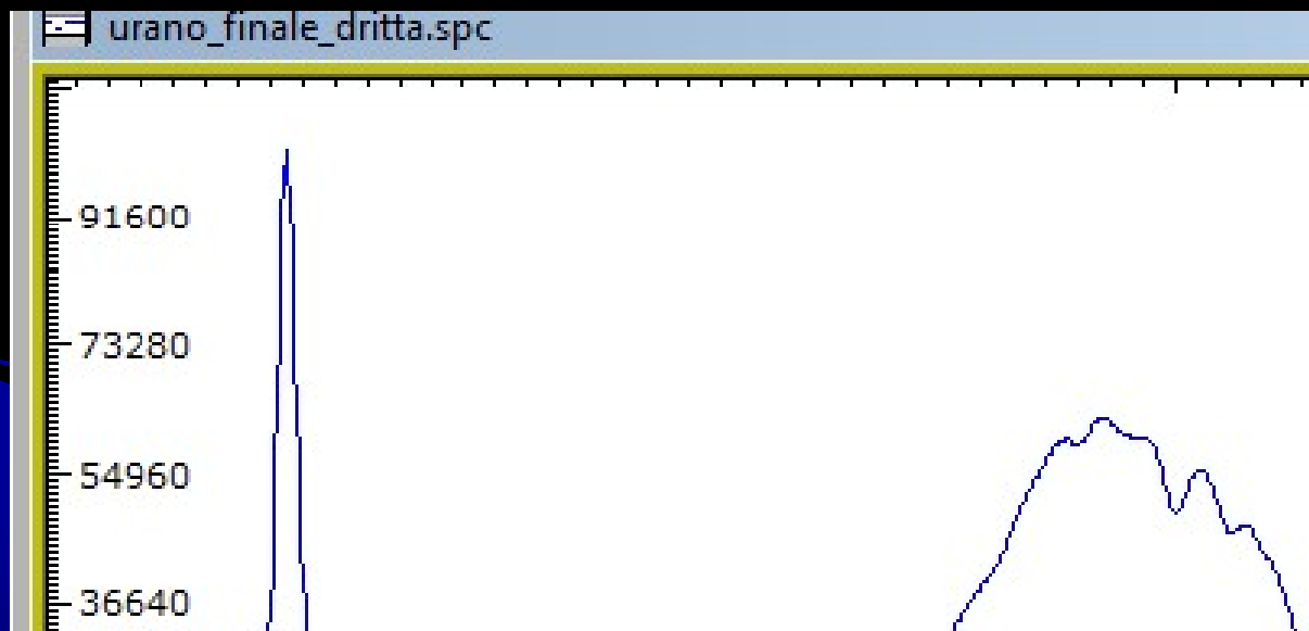
Profilo spettrale
